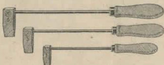
Lödkolv № K 99, av koppar med handtag av trä. Kolvens storlek 10×13×45 mm. Pris pr st. . . . . 0.45
