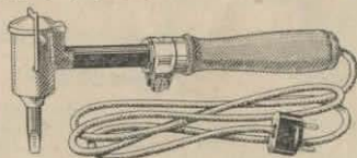
Elektrisk Lödkolv № K 105, strömförbrukning c:a 120 watt. För 110 eller 220 volt, för andra voltspänningar anskaffas på beställning. Med 180 cm. lång, gummiisolerad kabel o. stickkontakt, kolvens vikt med sladd c:a 600 gram. Pris . . . . . 12.50
