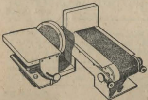
Ritning till en kombinerad band- & skivputsmaskin.
