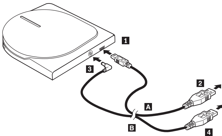
Abbildung 1-3. Konfiguration 3: Stromversorgung über USB-Standardbus
