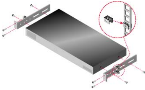
그림 2.2: 기기 수평 설치
