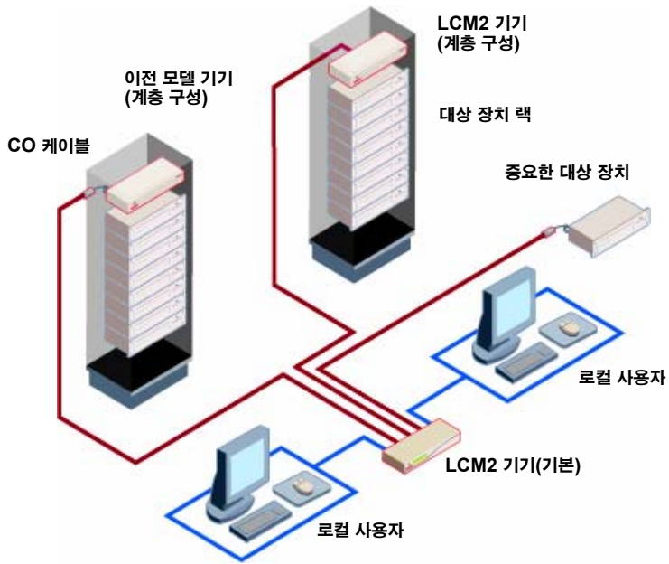
그림 1.3: LCM2 기기 구성의 예
