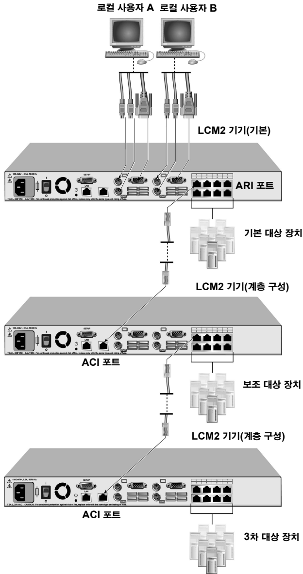
그림 2.4: 계층 구성된 기기를 포함하는 LCM2 기기 구성
