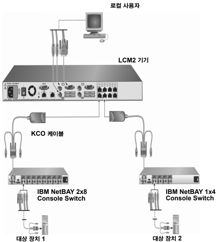
그림 2.5: 이전 모델 기기가 포함된 기기 구성
