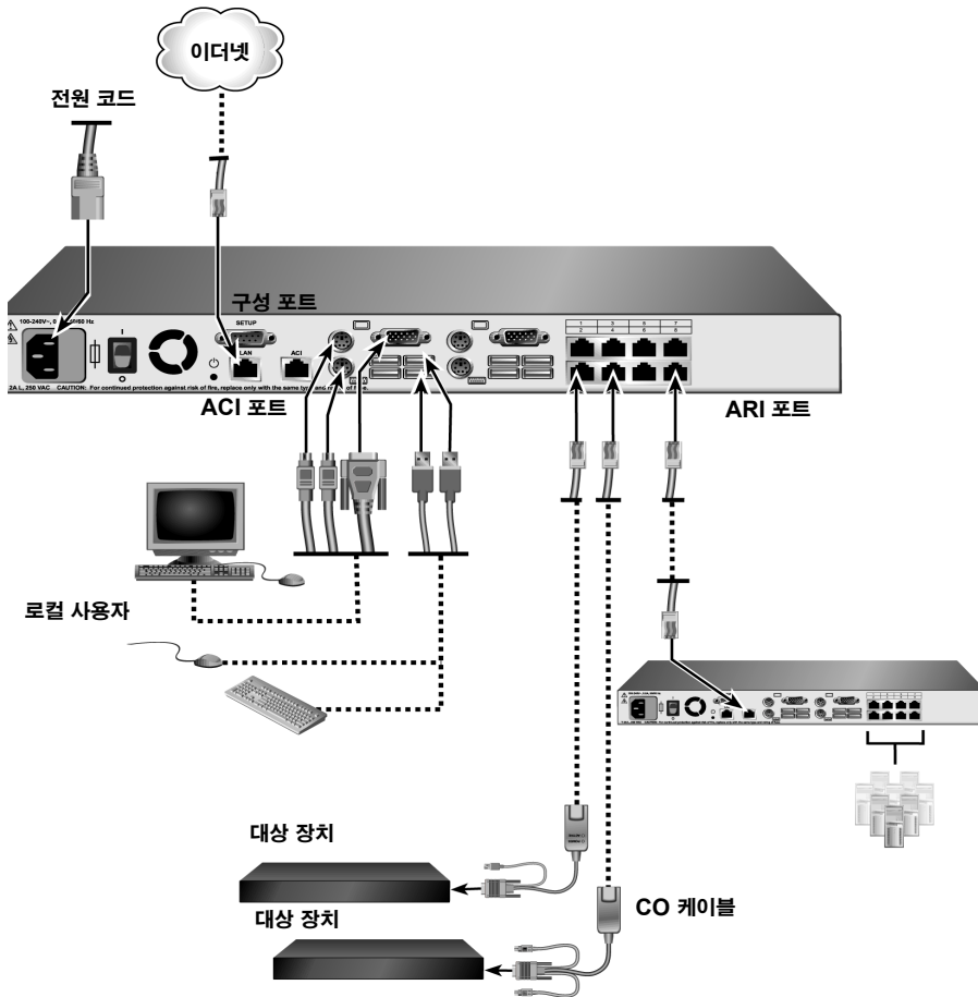
그림 2.3: 기본적인 LCM2 기기 구성
