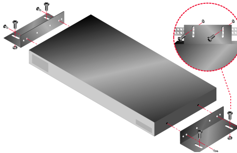
그림 2.1: 기기 수직 설치
