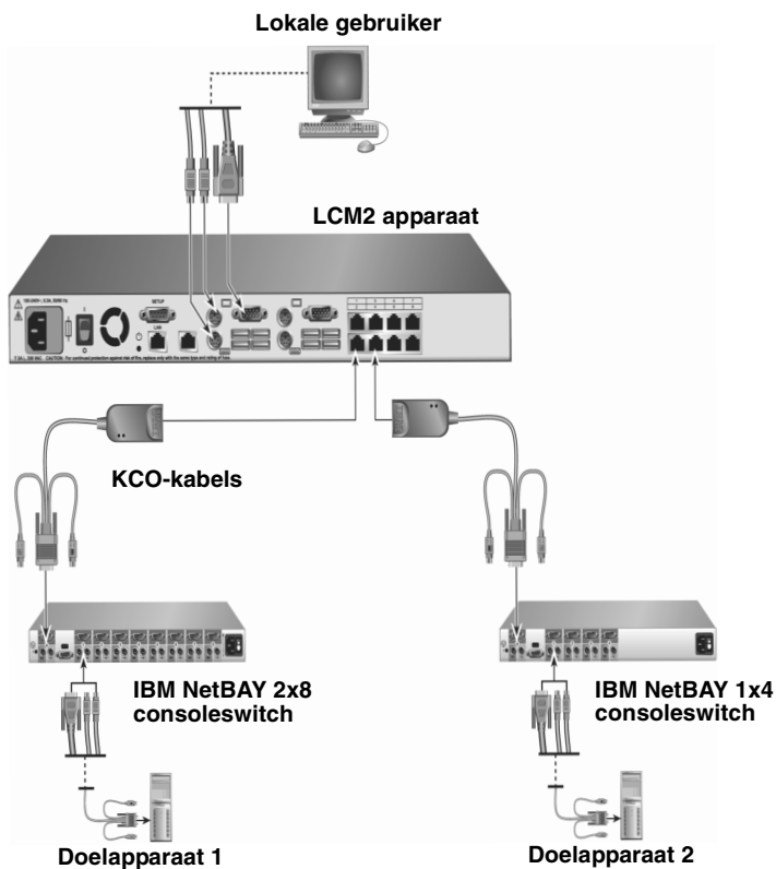
Afbeelding 2.5: Configuratie met toestellen van een ouder model
