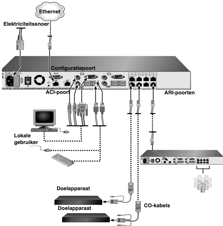
Afbeelding 2.3: Elementaire LCM2 apparaatconfiguratie
