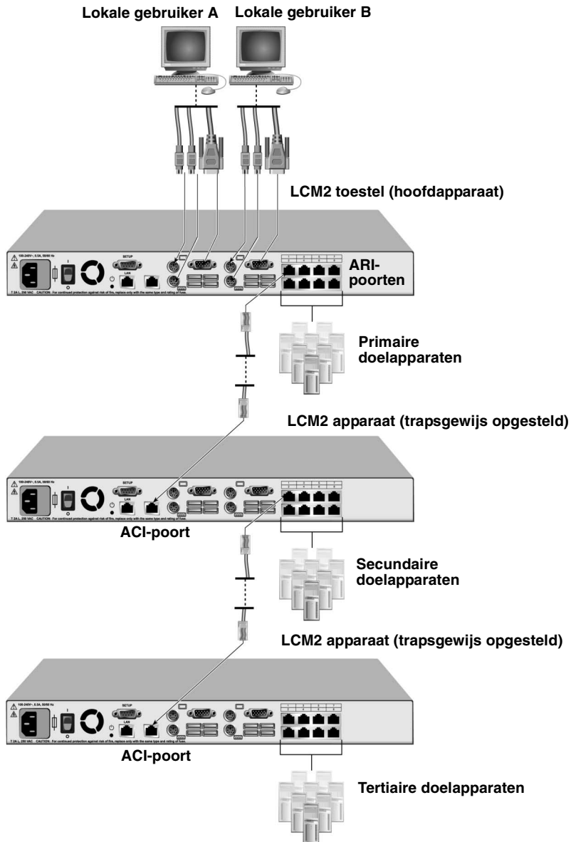
Afbeelding 2.4: Configuratie LCM2 met trapsgewijs opgestelde toestellen
