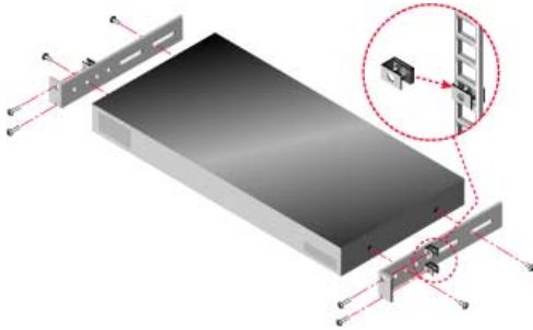
Afbeelding 2.2: Horizontale montage apparaat
