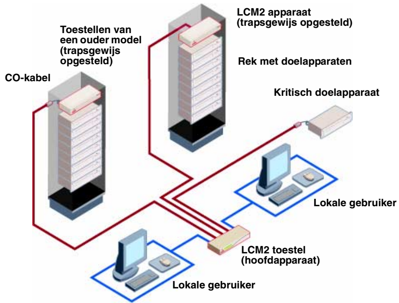
Afbeelding 1.3: Voorbeeld configuratie LCM2
