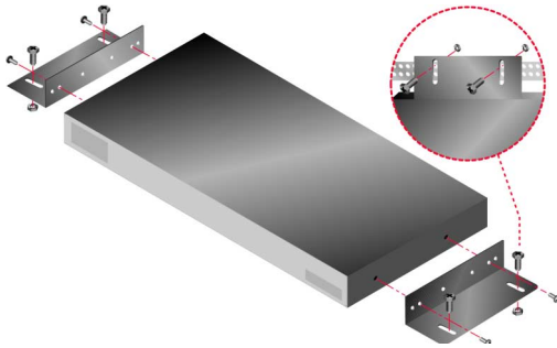
Afbeelding 2.1: Verticale montage apparaat
